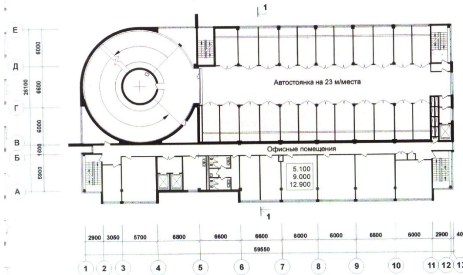
План на отм. 3.900, 6.900, 9.900, 12.900
