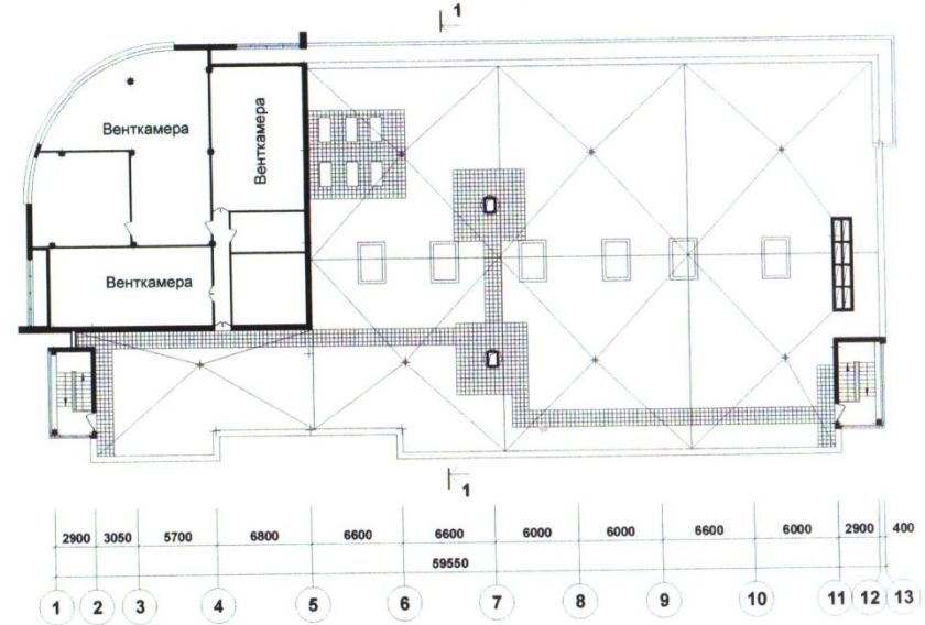
План на отм. 20.700
