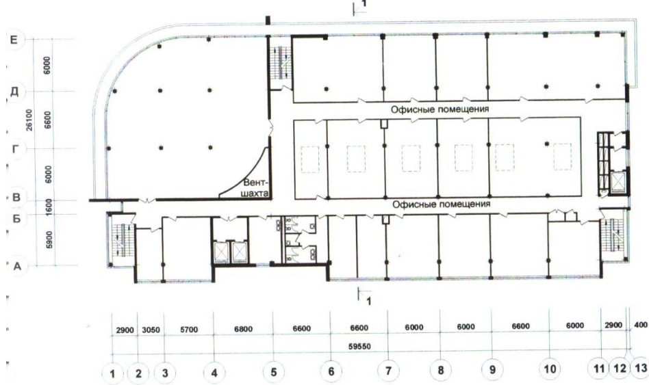
План на отм. 16.800
