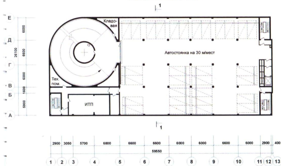
План на отм. -9.000, -6.000
