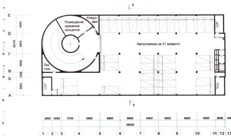
План на отм. -12.000
